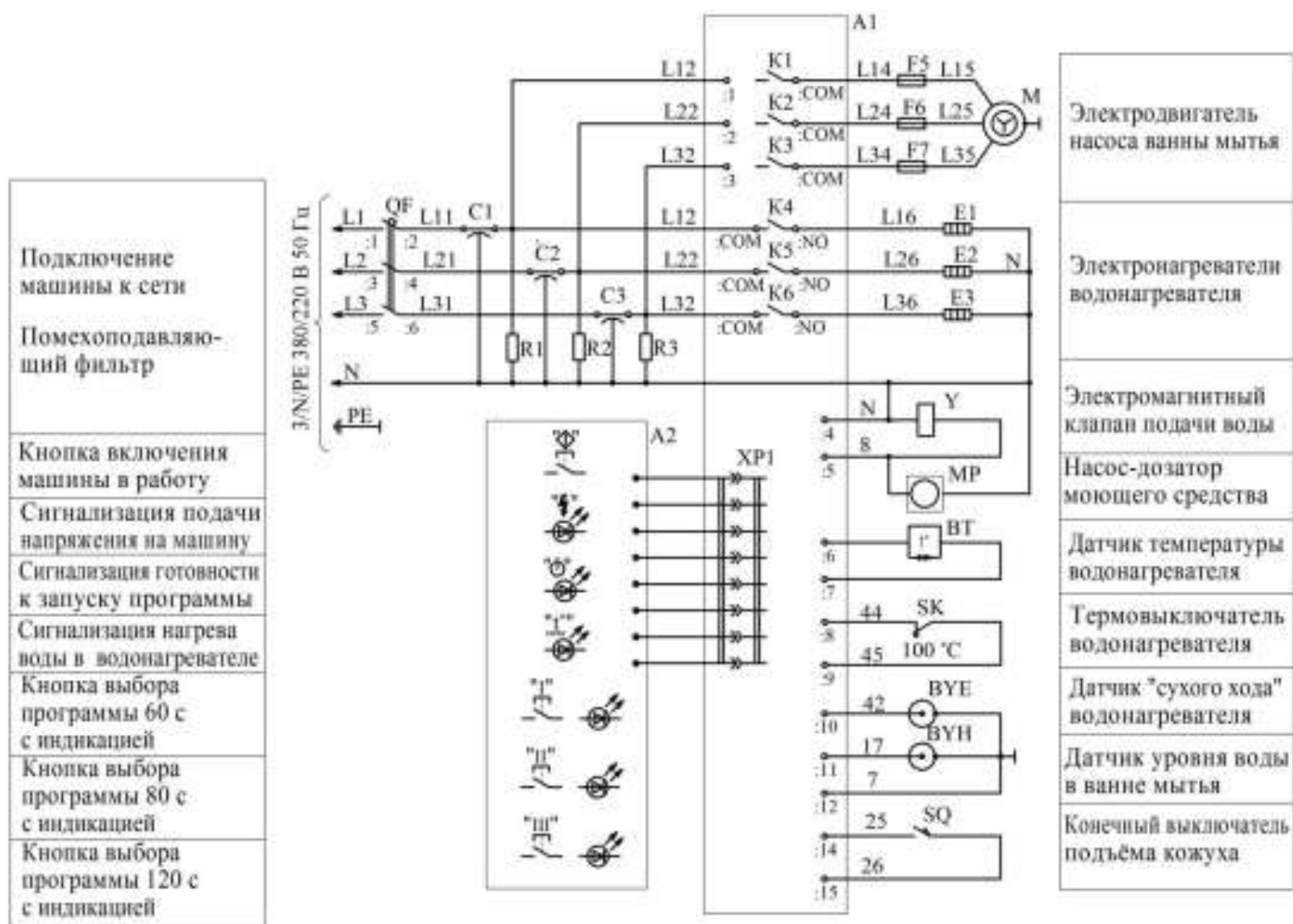
Рисунок 3 – Схема электрическая принципиальная
